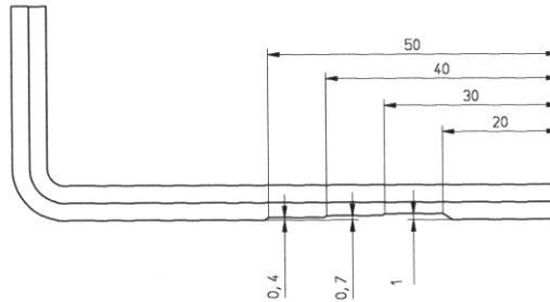
Abb. 8: Innensechskantschlüssel mit Einkerbungen
