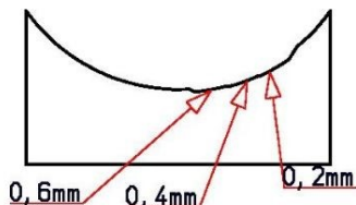
10. sz. ábra: Vágási mélységek a késbeállító eszközön
