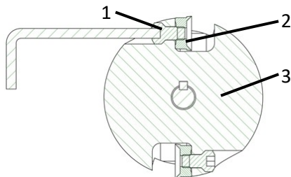
16. sz. ábra: A kések cseréje
