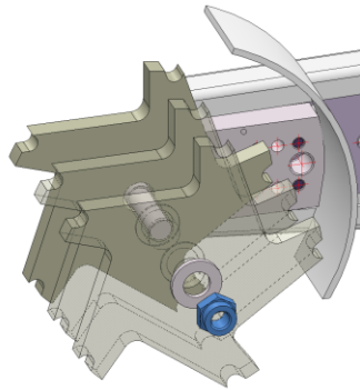
Abb. 12: Messer wechseln an der Nutenfräse
