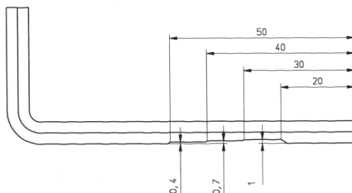
Fig. 8 : Clé Allen avec encoches
