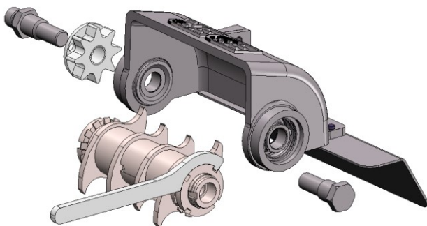
Obr. 14: Výmena nožov
