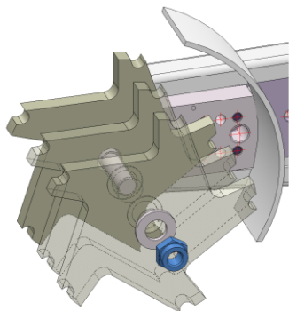
Fig. 12: Cambio dei coltelli sulla fresatrice scanalatrice
