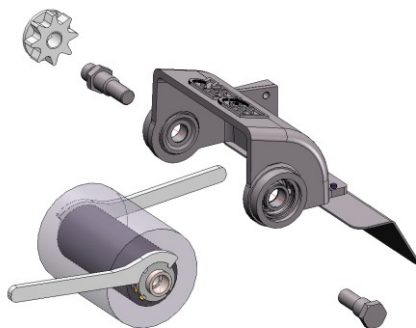
Fig. 13: Cambio della spazzola rotante
