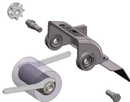
Obr. 13: Výmena okrúhlej kefy
