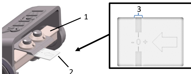
Obr. 7: Nastavenie noža
