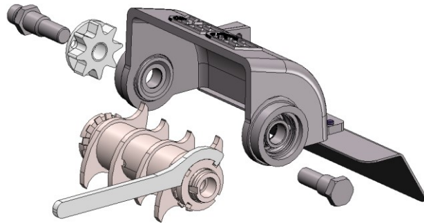
Abb. 14: Messer wechseln
