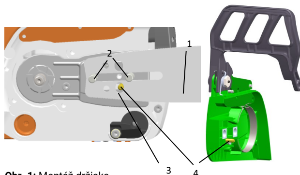
Obr. 1: Montáž držiaka
