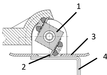
Obr. 9: Nastavení nožů
