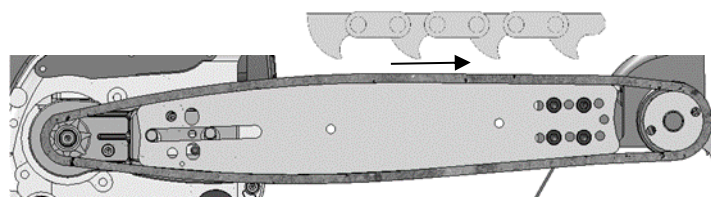
Obr. 3: Instalace řetězu
