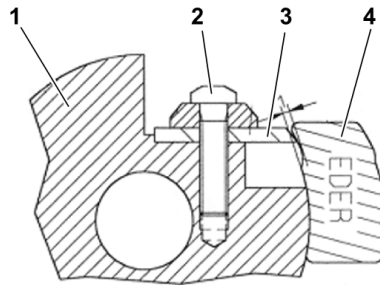
Obr. 15: Výměna nožů na kotoučové fréze
