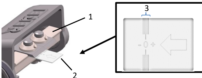
Obr. 7: Nastavení nožů
