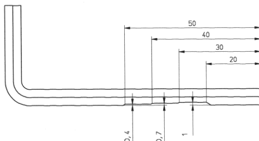
8. sz. ábra: Imbuszkulcs rovátkákkal
