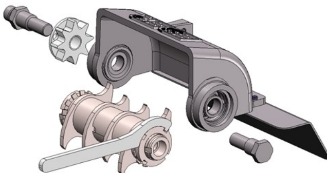
Obr. 14: Výměna nožů
