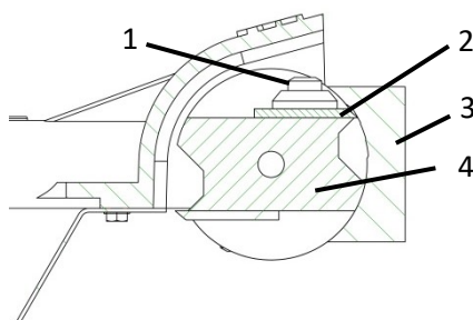
Obr. 11.: Nastavení nožů
