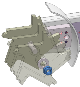
Obr. 12: Výmena nožov na drážkovacej fréze
