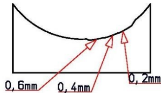
Abb. 10: Schnitttiefen an der Messerlehre
