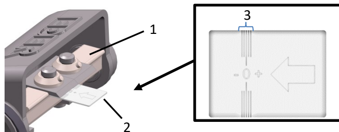
7. sz. ábra: A kés beállítása
