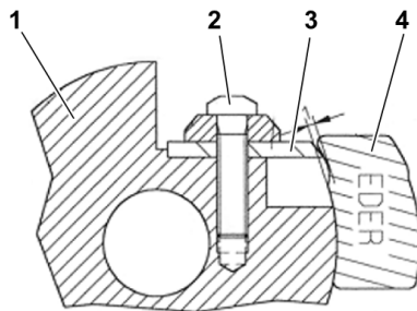
15. sz. ábra: Késcsere a tárcsamaron
