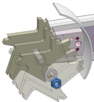
Fig. 12 : Remplacement des couteaux sur la fraiseuse rainureuse
