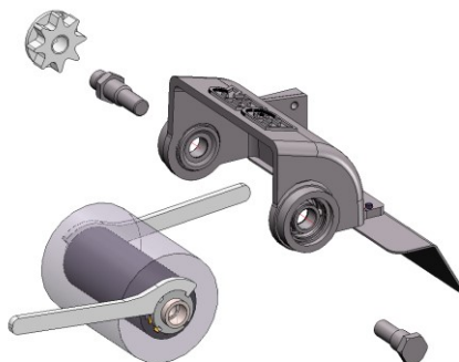
Fig. 13 : Remplacement de la brosse rotative
