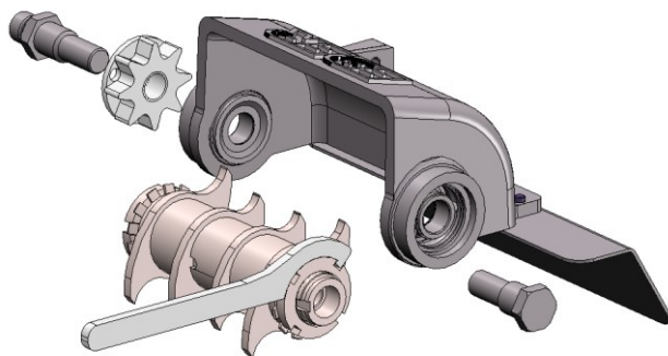
Fig. 14: Cambio dei coltelli
