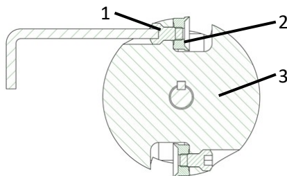
Obr. 16: Výmena nožov
