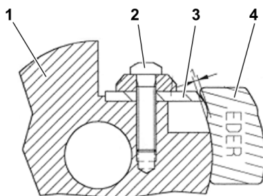
Obr. 15: Výmena nožov na kotúčovej fréze
