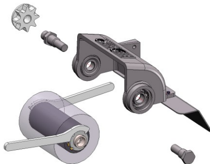
13. sz. ábra: A drótkefe cseréje
