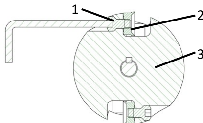
Fig. 5: Remplacement des copeaux
