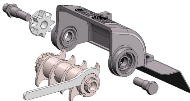
Fig. 14 : Remplacement des couteaux
