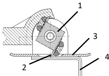
9. sz. ábra: A kés beállítása
