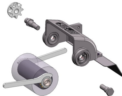
Abb. 13: Rundbürste wechseln
