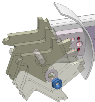
12. sz. ábra: A horonymaró kés cseréje
