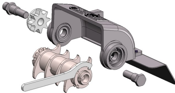
14. sz. ábra: A kések cseréje
