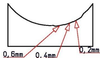
Fig. 10: Taglio di profondità sul calibro del coltello
