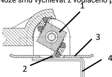
Obr. 9: Nastavenie noža
